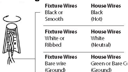
Fig. 3 Wiring
