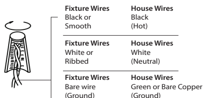
Fig. 2 Wiring
